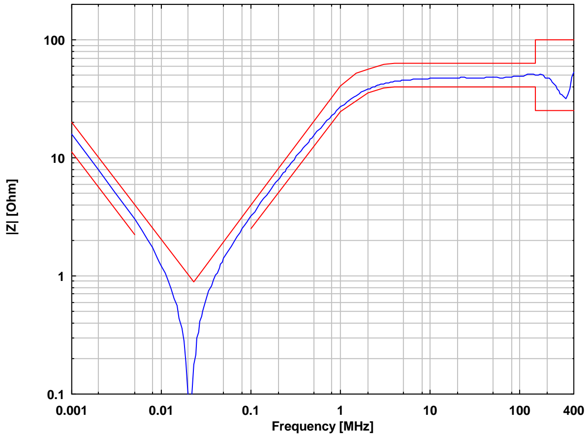
Abb. 9: Betrag der Impedanz an den Prüflingsklemmen nach DEF STAN 59-411 (Kalibrieradapter KA 8125 erforderlich), BNC mit 50 \Omega Abschluss, 10 \mu\text{F} Kondensator an den Speiseklemmen Fig. 9: Magnitude of impedance at EuT-Terminals in acc. to DEF STAN 59-411 (Calibration adapter KA 8125 required), BNC-Port terminated with 50 \Omega , 10 \mu\text{F} Capacitor across mains terminals
