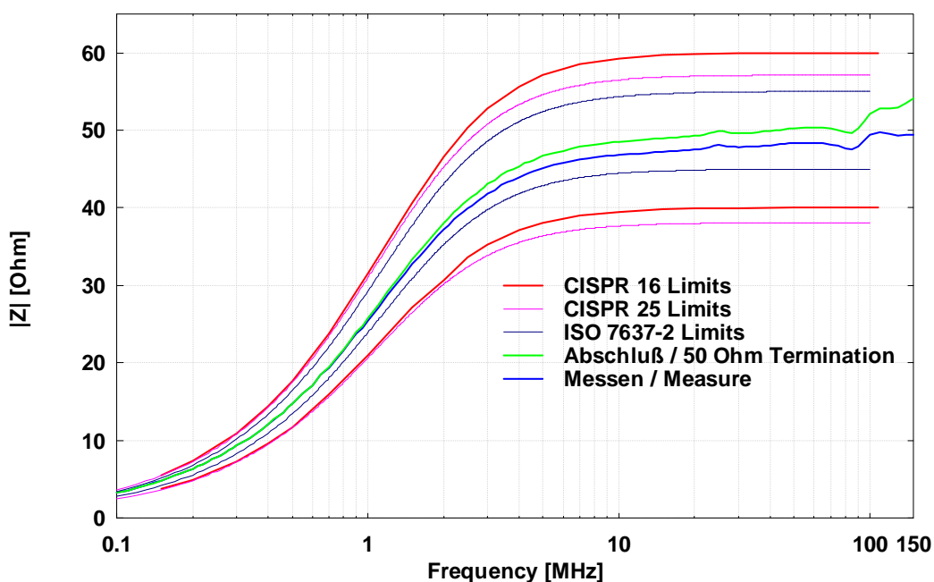
Abb. 4: Betrag der Impedanz an den Prüflingsklemmen (Kalibrieradapter KA 8125 erforderlich), BNC mit 50 Ω Abschluss, Speiseklemmen kurzgeschlossen
