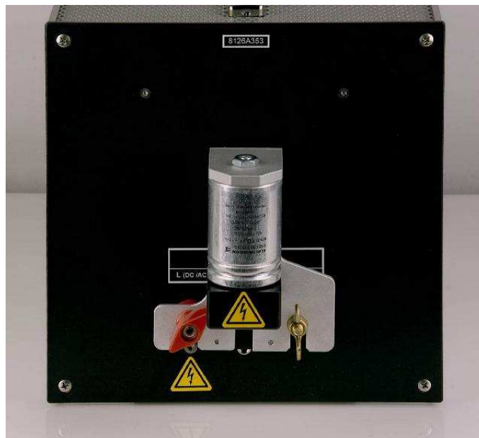
Abb. 3: Befestigung des CAP 10 an einer Netznachbildung Fig. 3: CAP 10 mounted to a LISN
